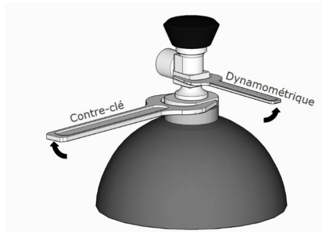
Figure 3. Utilisation de la contre-clé pour le démontage de la vanne.
