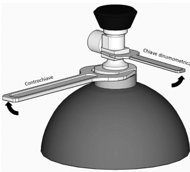
Figura 3. Uso della controchiave per smontaggio della valvola
