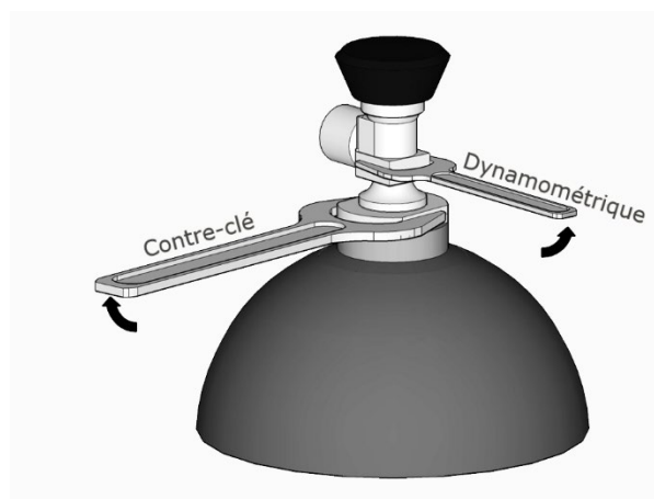
Figure 3. Utilisation de la contre-clé pour le démontage de la vanne.
